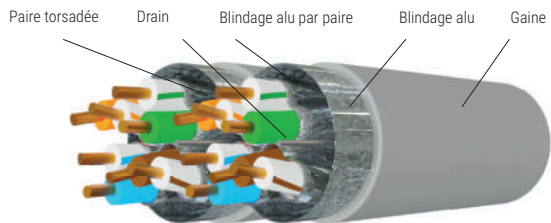
F/FTP
