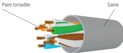
U/UTP
