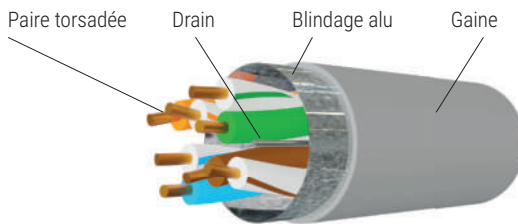
F/UTP
