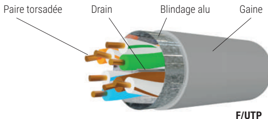
F/UTP
